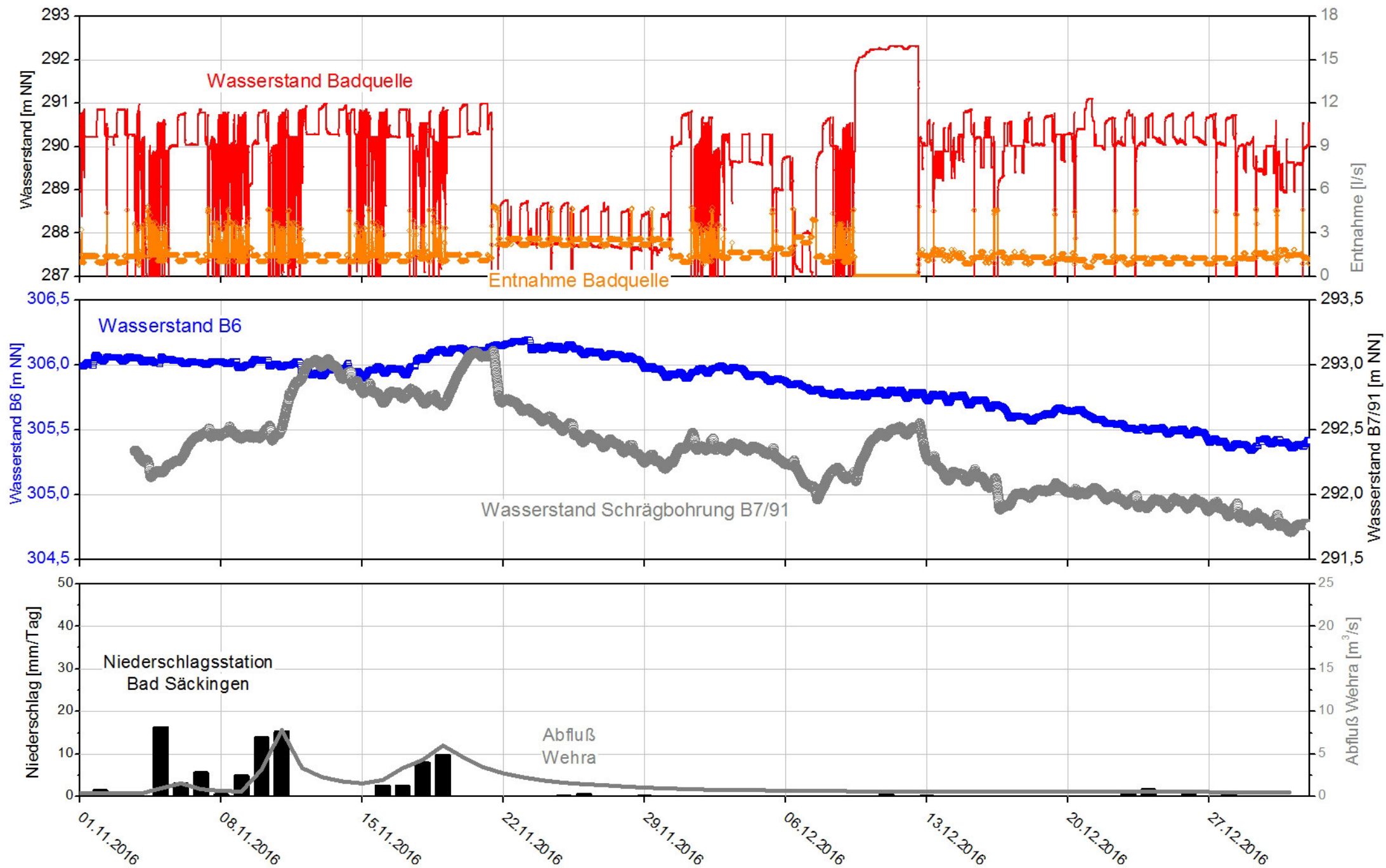
Anl. 4b: Vergleichende Darstellung zu den Wasserständen an der Badquelle und umgebender Aufschlüsse (Zeitraum 11-12.2016)
