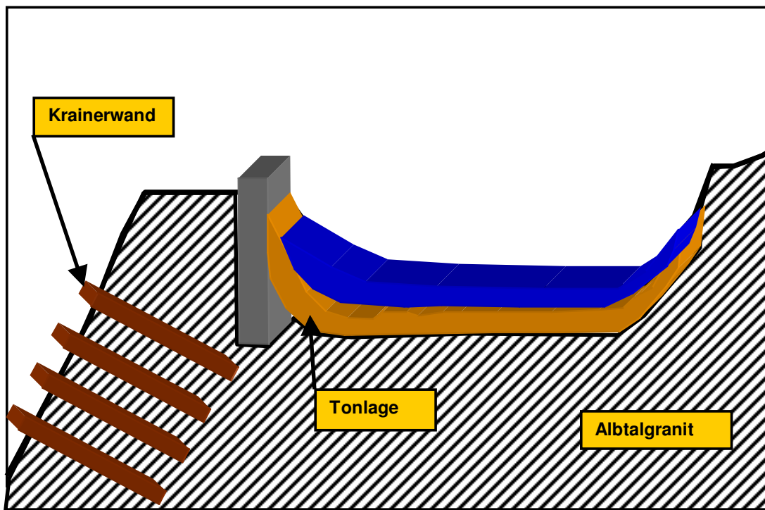
Abb. 16: Abdichtung des Heidenwuhes mit einer Tonlage.
