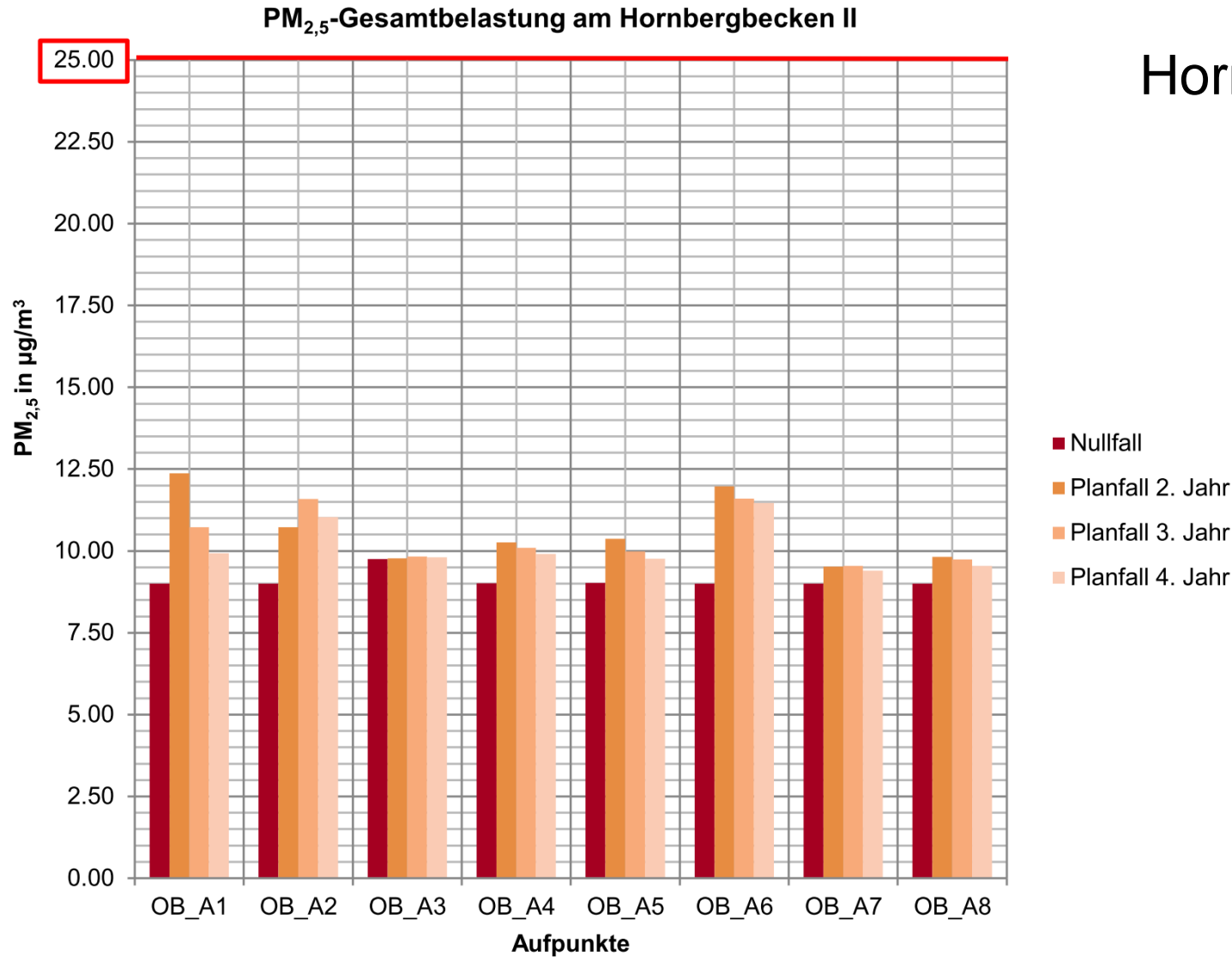
Abbildung 9-3: PM 2,5 -Gesamtbelastung im Nullfall und Planfall am Hornbergbecken II an den Aufpunkten in µg/m 3 (Grenzwert 25 µg/m 3 ).
