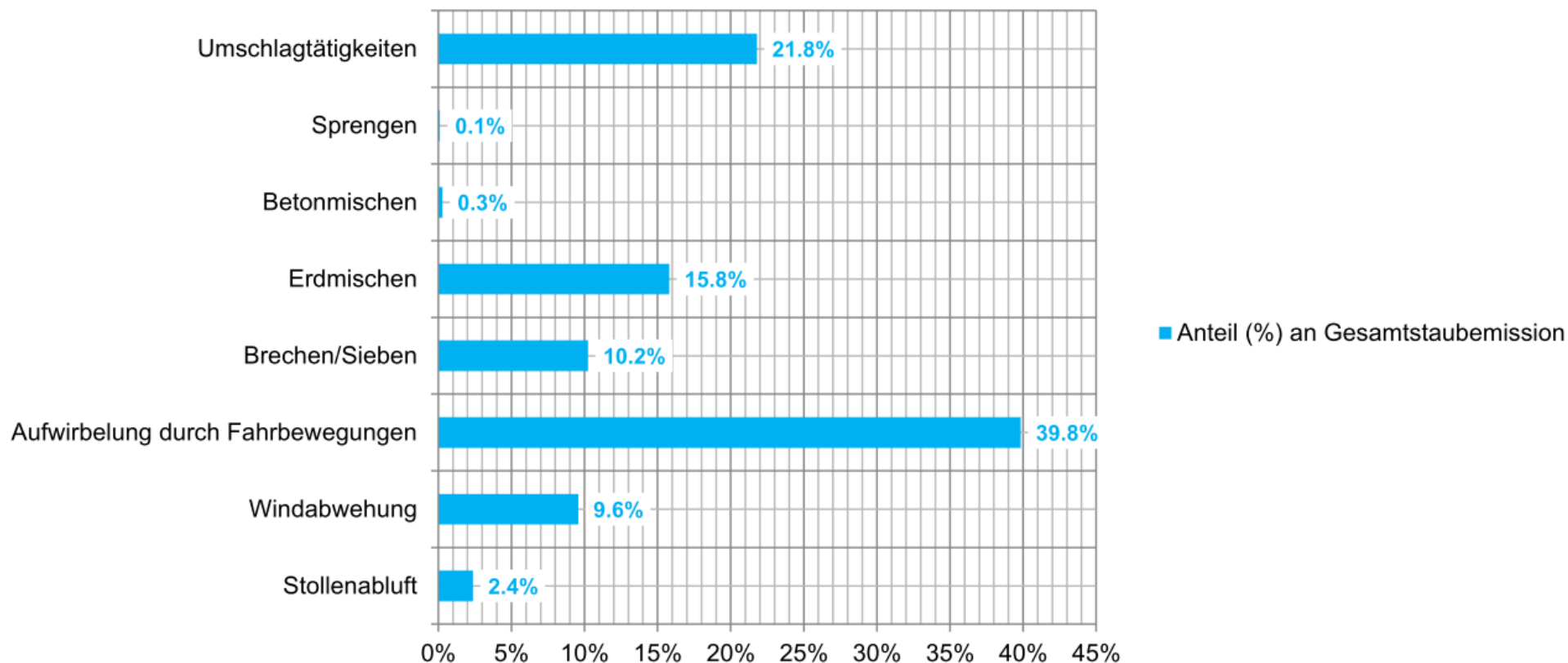
Prozentuale Anteile der staubemittierenden Prozesse am HBBII im 2. Jahr
